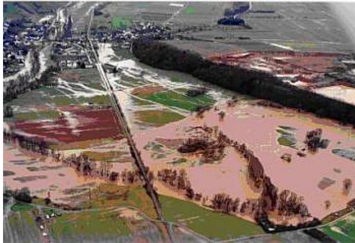
Foto von der Lieser, Ortslage Platten, beim Hochwasser am 03.01.03. Das Bild verdeutlicht die Überflutungssituation einige Stunden nach dem Höchststand, d.h. bei bereits fallendem Wasserstand
